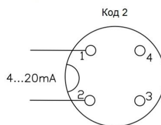
M12 4pin
