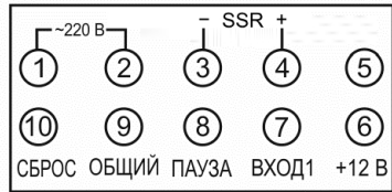
Рис. 7 Схема подключения ARCOM-TC-D44 с SSR
