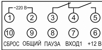
Рис. 6 Схема подключения ARCOM-TC-D44 с реле
