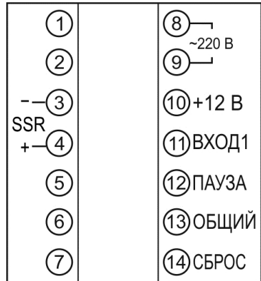
Рис. 9 Схема подключения ARCOM-TC-D77 с SSR
