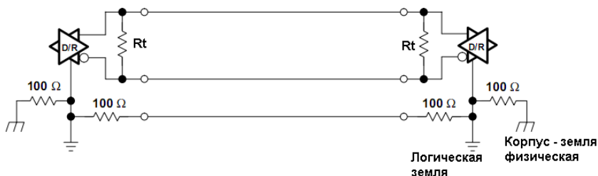
Рис. 2.2 Структура сети RS485 с заземлением
