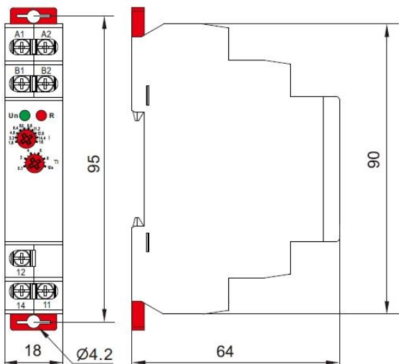
Рис. 3 – Размеры прибора
