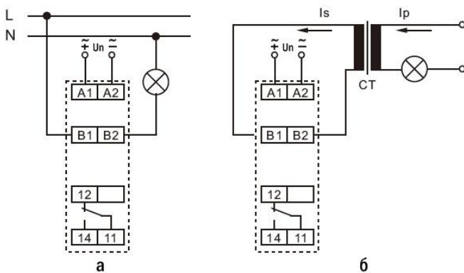
Рис. 2 – Схема подключения
