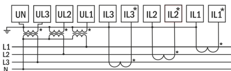
Рис. 8 – Подключение трансформаторов тока и напряжения
