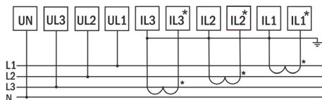
Рис. 6 – Подключение трансформаторов тока
