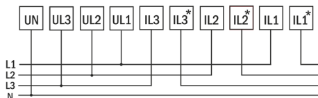
Рис. 5 – Подключение напрямую
