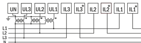
Рис. 7 – Подключение трансформаторов напряжения
