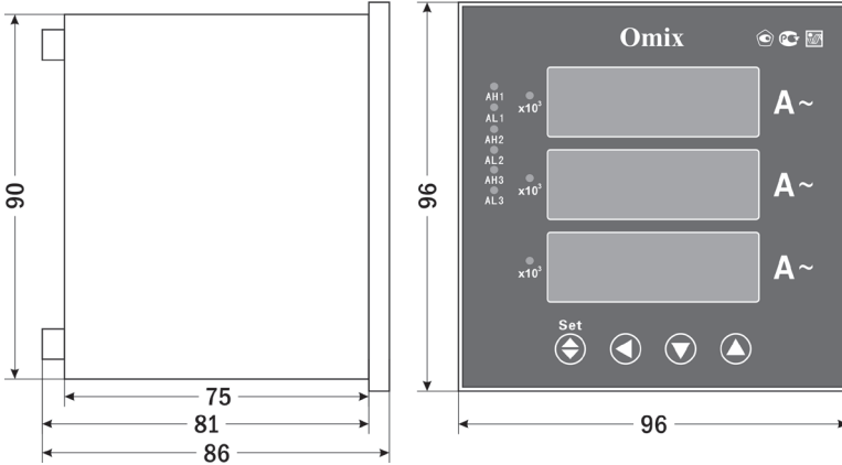
Рис. 3 – Размеры прибора
