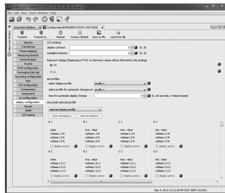
Рис. Настройка профиля в программе GridVis.
