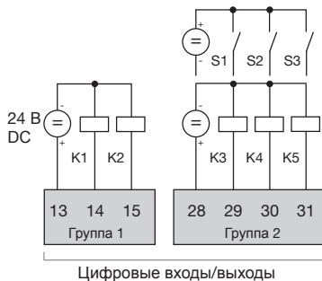
Рис.: Цифровые входы группы 1 и цифровые входы/выходы группы 2
