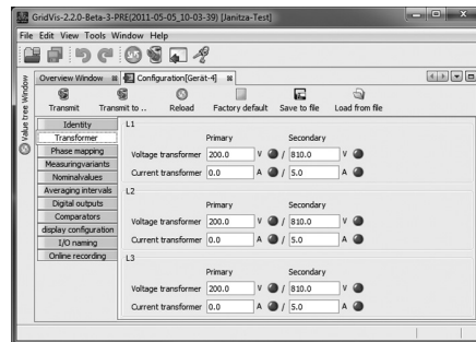
Рис. Раздел настройки трансформаторов тока и напряжения в программе GridVis.
