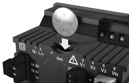
Рис. Слот для батареи с обратной стороны
