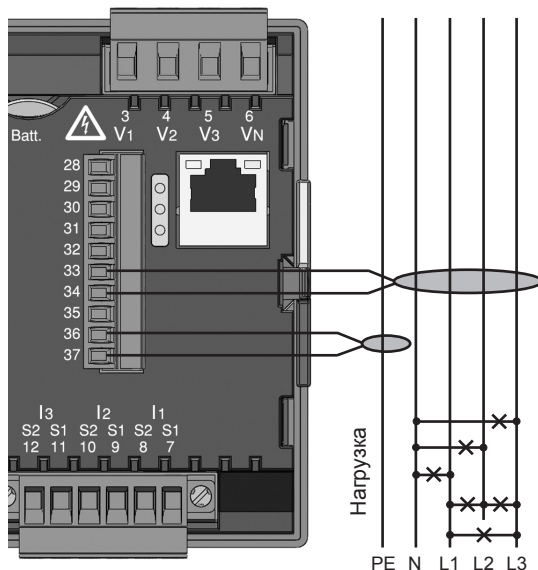
Рис. Пример подключения, измерение дифференциального тока через трансформатор тока
