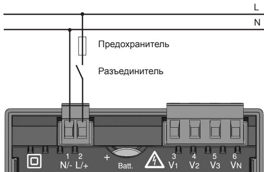
Рис. Пример подключения питания к UMG 96RM
